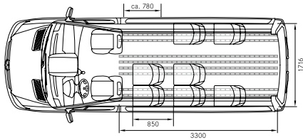
Sprinter Mobility 23, Bestuhlungsvariante 7 + 1 + 1 Sitzplätze
