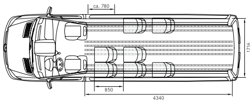
Sprinter Mobility 33, Bestuhlungsvariante 7 + 1 + 1 Sitzplätze
